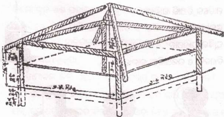
ଶସ୍ତ୍ରା କୁକୁଡ଼ା ଘର ନକ୍ସା
